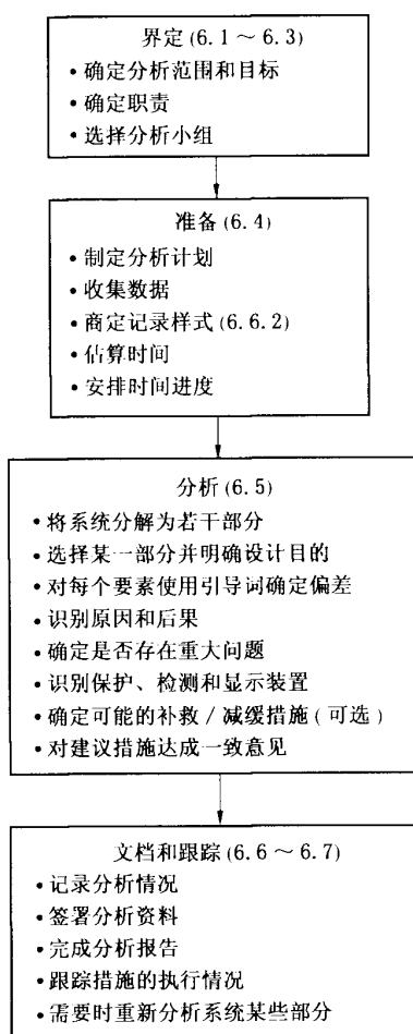
图 1 HAZOP 分析程序
