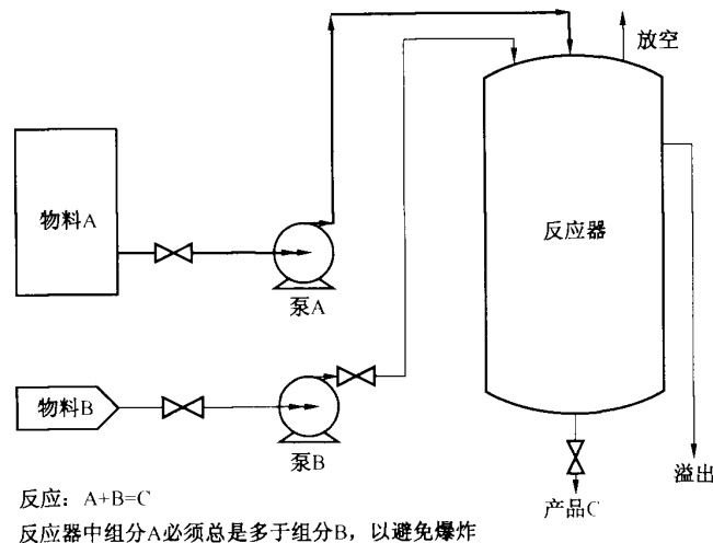
图 B.1 简化流程
