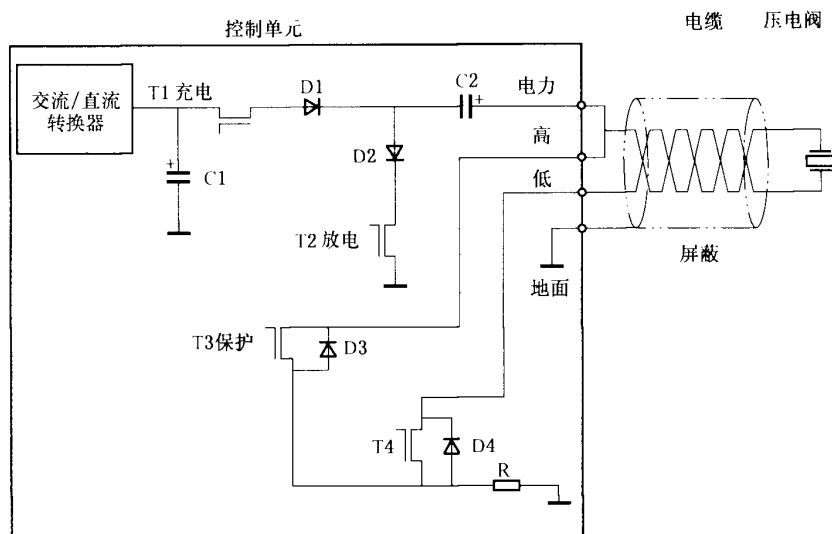
图 B.3 压电阀控制系统
