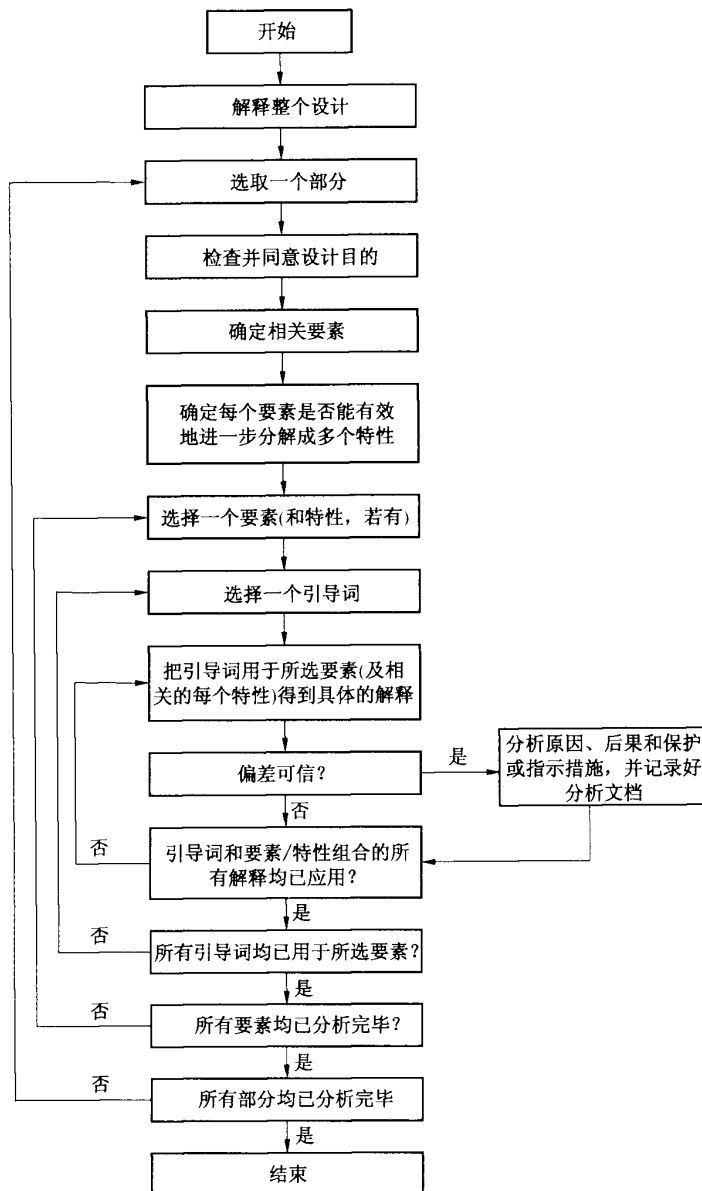
图2 HAZOP分析程序流程——要素优先顺序
