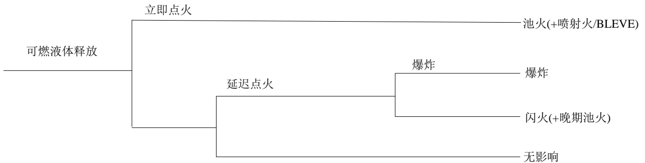
图 G.5 可燃液体释放事件树
