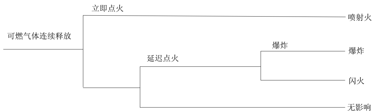
图 G.2 可燃气体连续释放事件树
